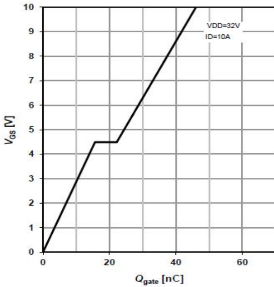
Typ.gate charge
