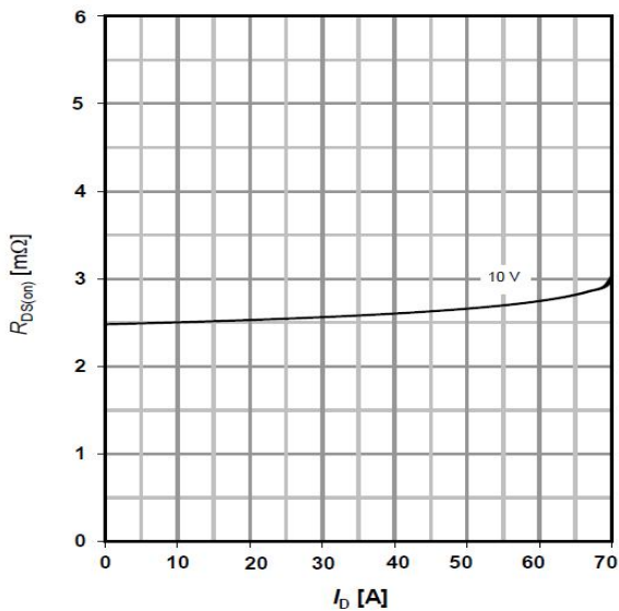
RDS(on) -- ID
