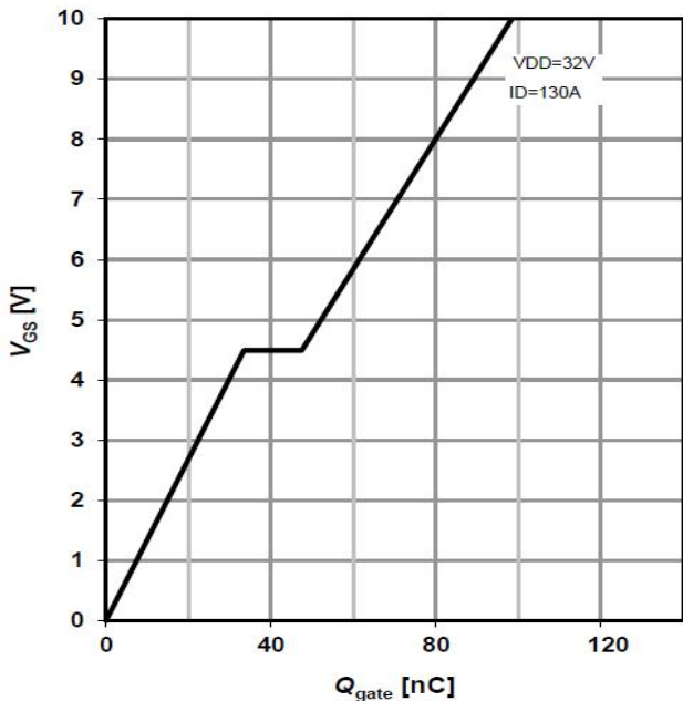
Typ.gate charge
