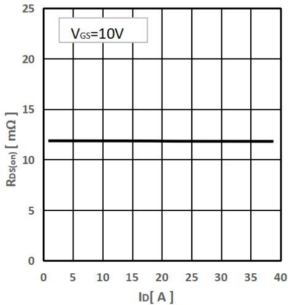
RDS(on) -- ID
