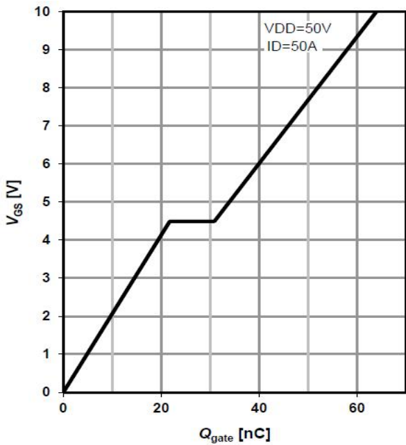
Typ.gate charge
