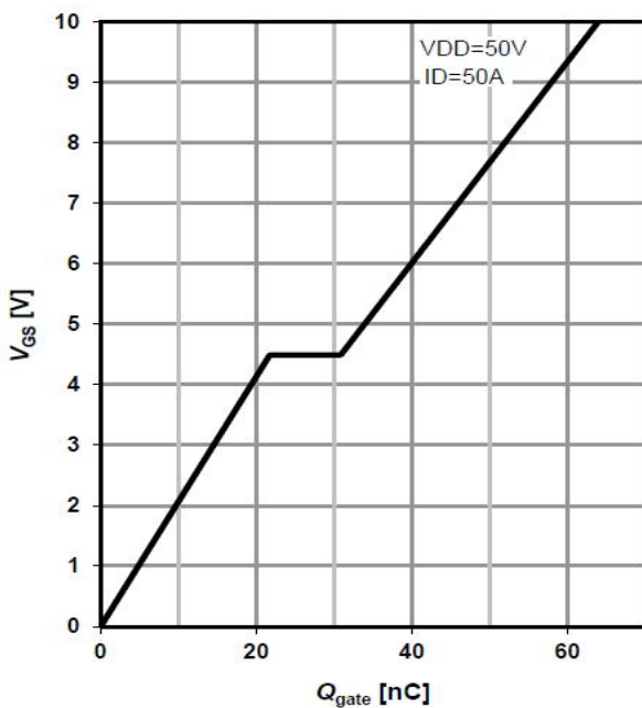
Typ.gate charge
